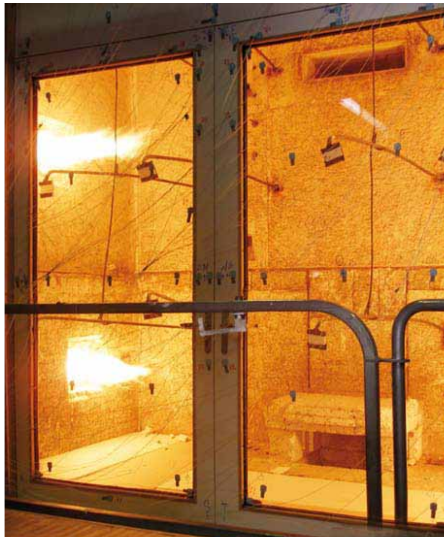
Prüfung des Brandverhaltens nach DIN EN 1634-1.
