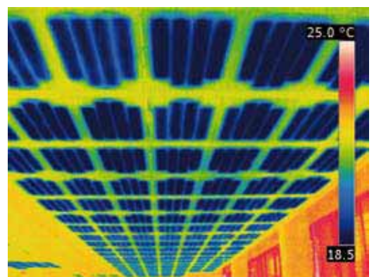
Thermografie zur Prüfung der Funktionstüchtigkeit von Kühldecken
